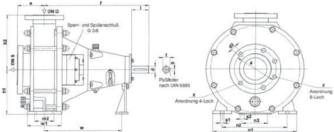
Maßbild, Pumpekopf / Lagerträger kpl.
